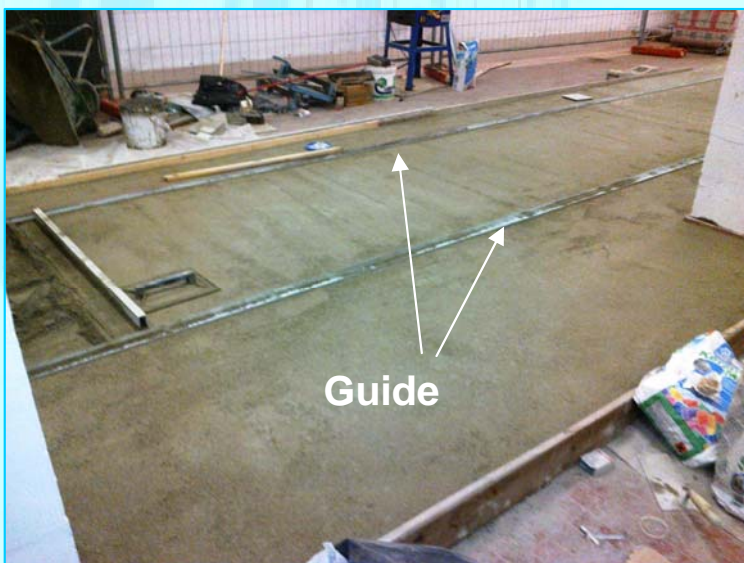
Livellamento della pavimentazione mediante basamenti in c.a.
