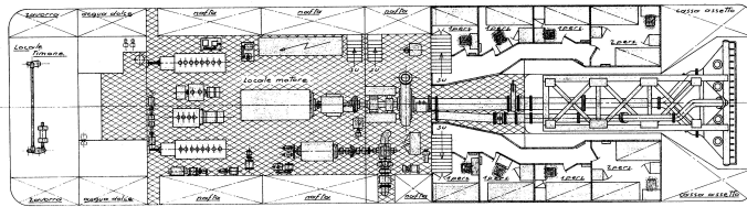
PIANO DI MACCHINA E ALLOGGI
